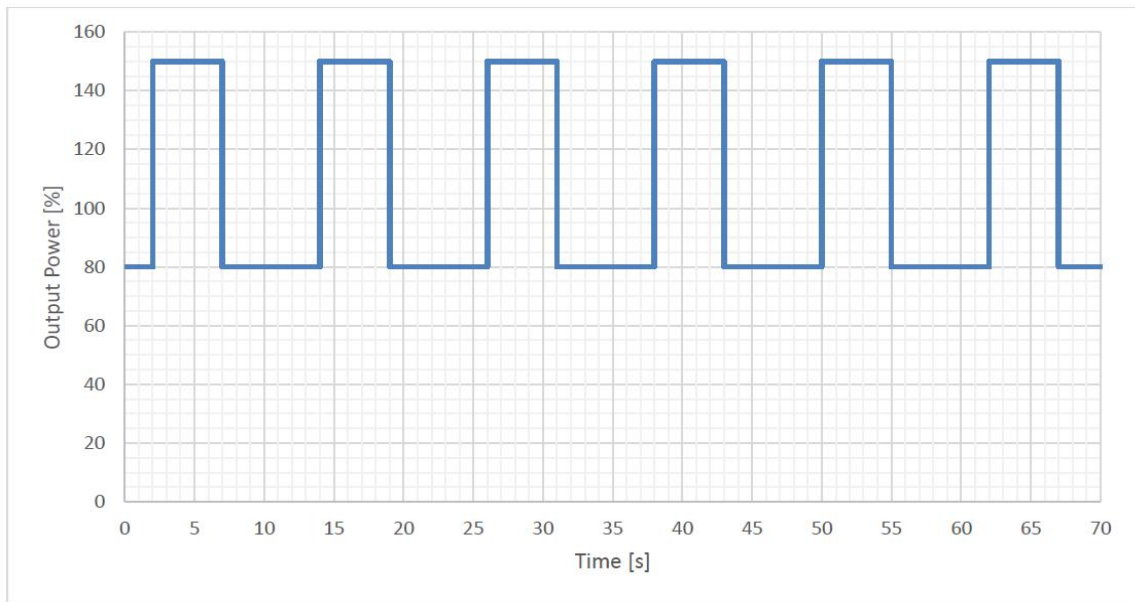
图1: 环温50℃情况下 (80%→150%输出功率) , 峰值功率时间5s
