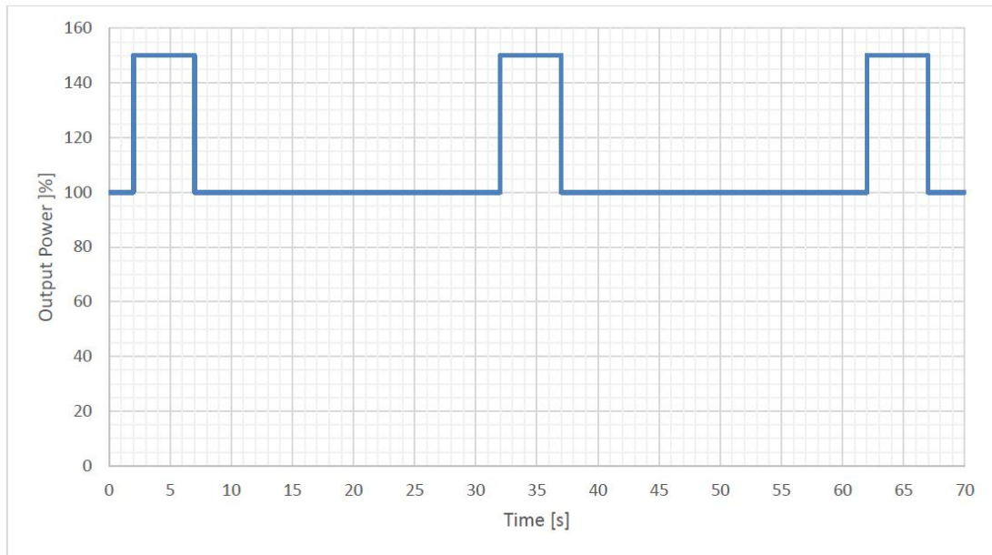
图2: 环温50℃情况下 (100%→150%输出功率) , 峰值功率时间5s
